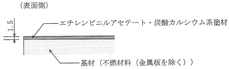
図1 断面図
